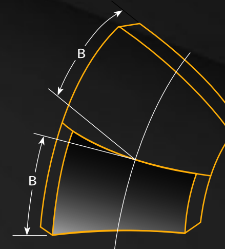
Codo 45°
