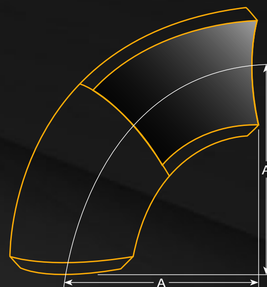
Codo 90° R.L.
